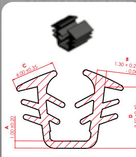
EXTRUEMPAQUE UNIVERSAL 3-4 MM C030300
