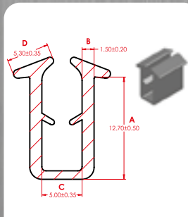
EMPAQUE EN U PARA VIDRIO FIJO 6 MM C030106
