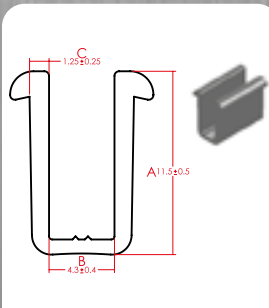
EMPAQUE EN U PARA VIDRIO FIJO 4 MM C030021
